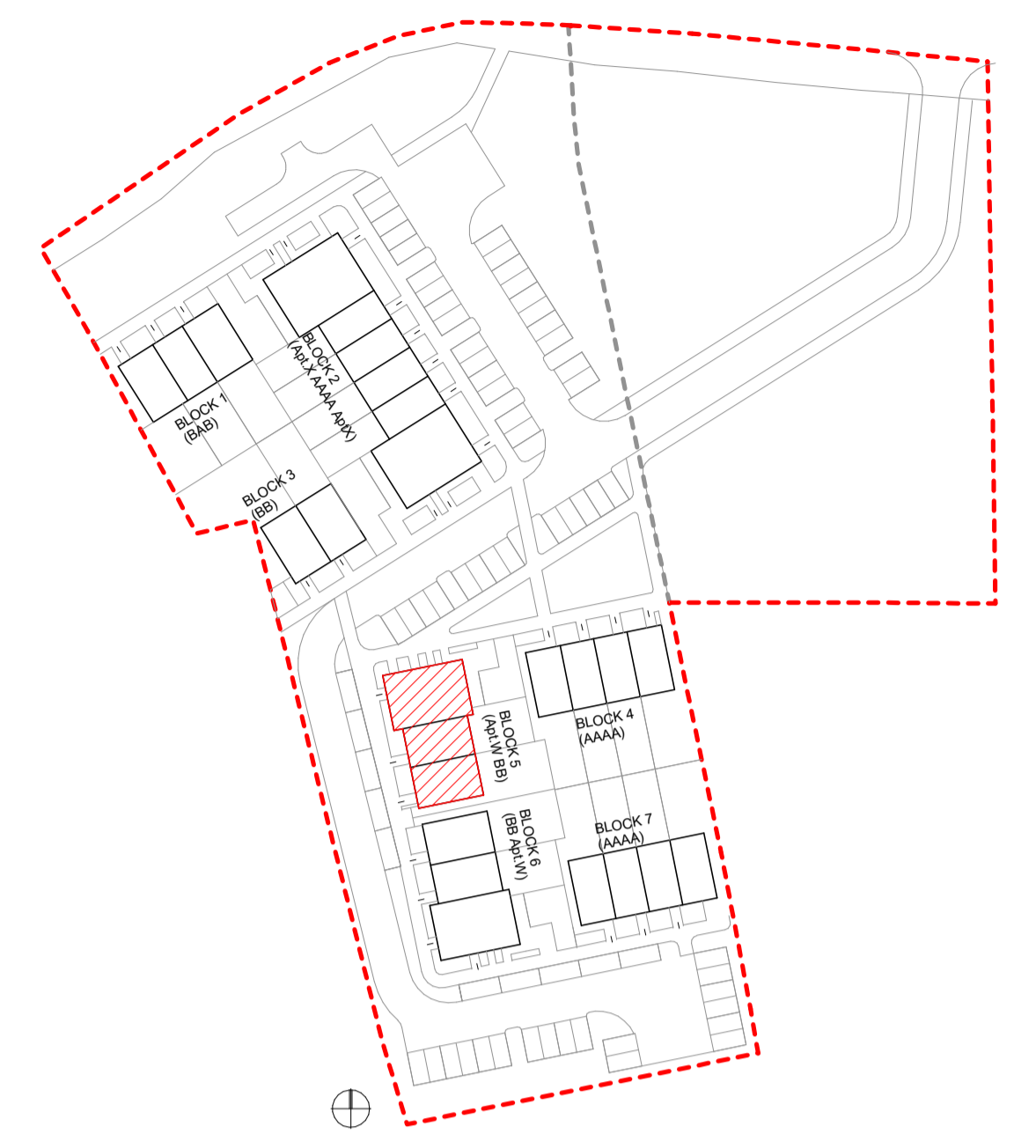
Key Plan 1 : 1000
